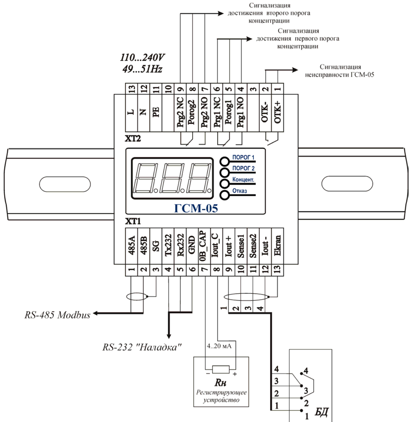
Схема подключения ГСМ-05
