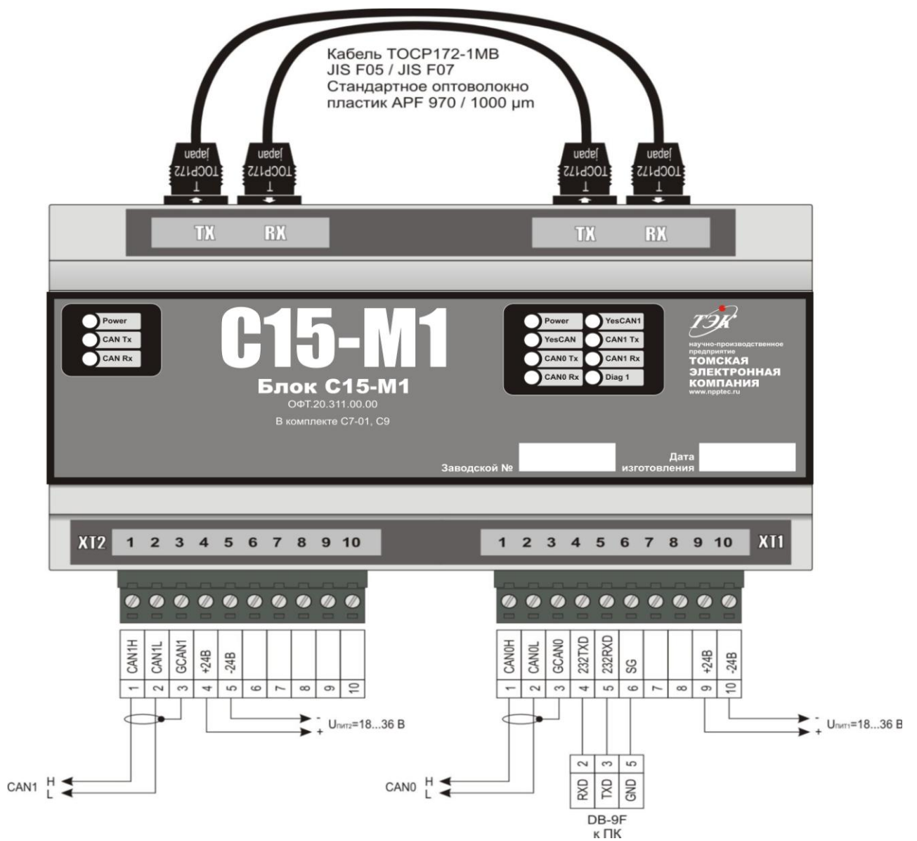
Рисунок 2 - Схема внешних подключений
