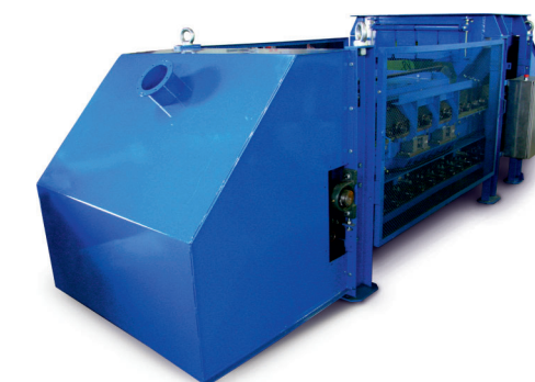
Дозатор пластинчатый непрерывного действия (температура материала до 600°C)
