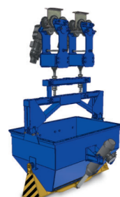
Тележка транспортная монорельсовая ТТМ
