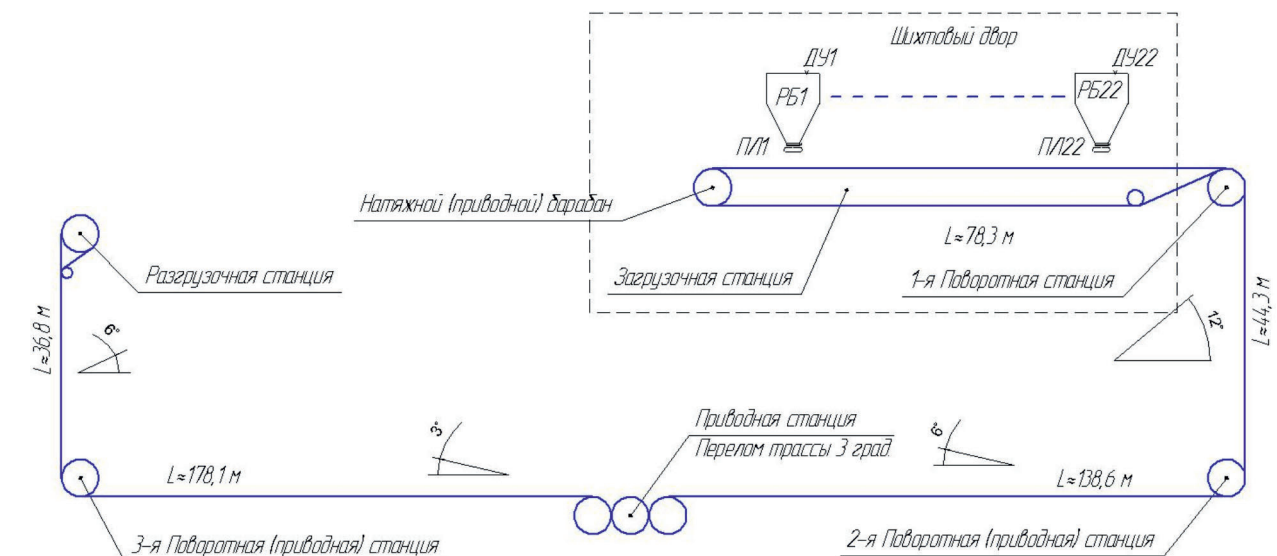
Трасса конвейера «SICON» - дублирующий тракт
