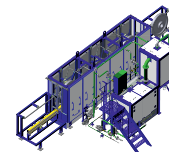
Установка подготовки поверхности с вертикальной загрузкой
