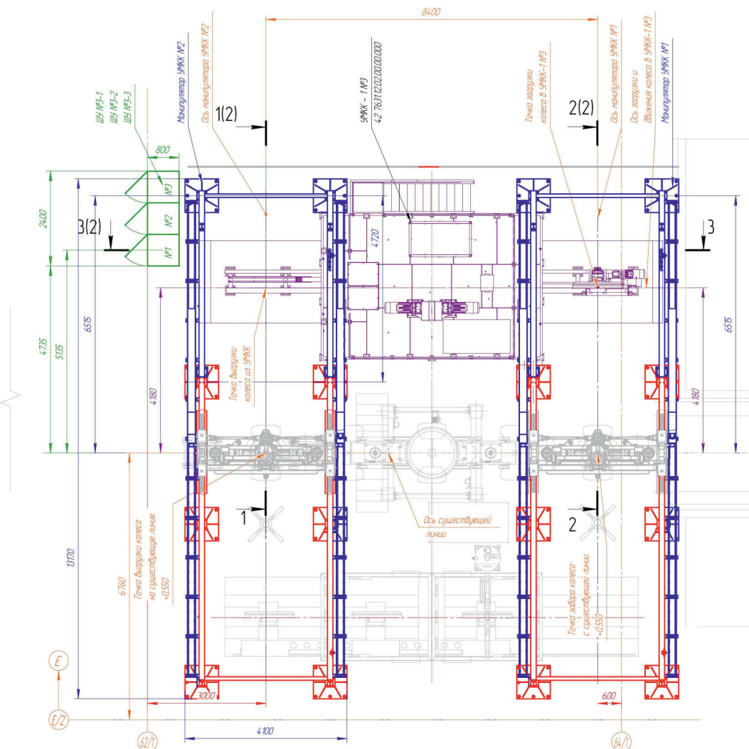
Планировка ЛВК №2
