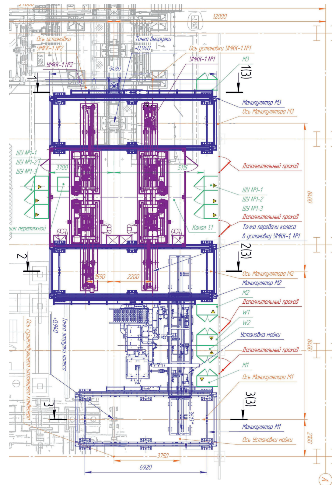
Планировка ЛВК №1
