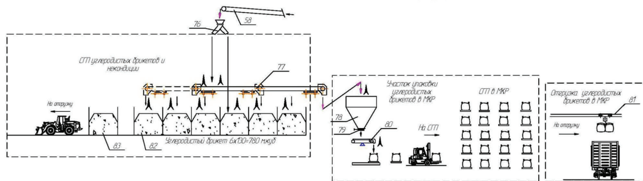
Склад готовой продукции
