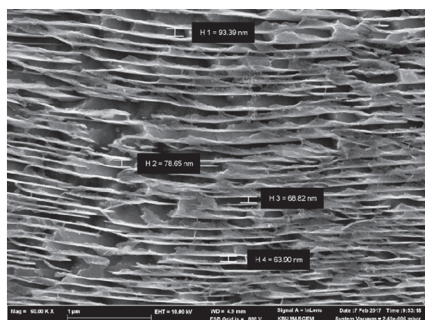
Микроструктура головки рельсов термообработанной по технологии ТЕС-DT
